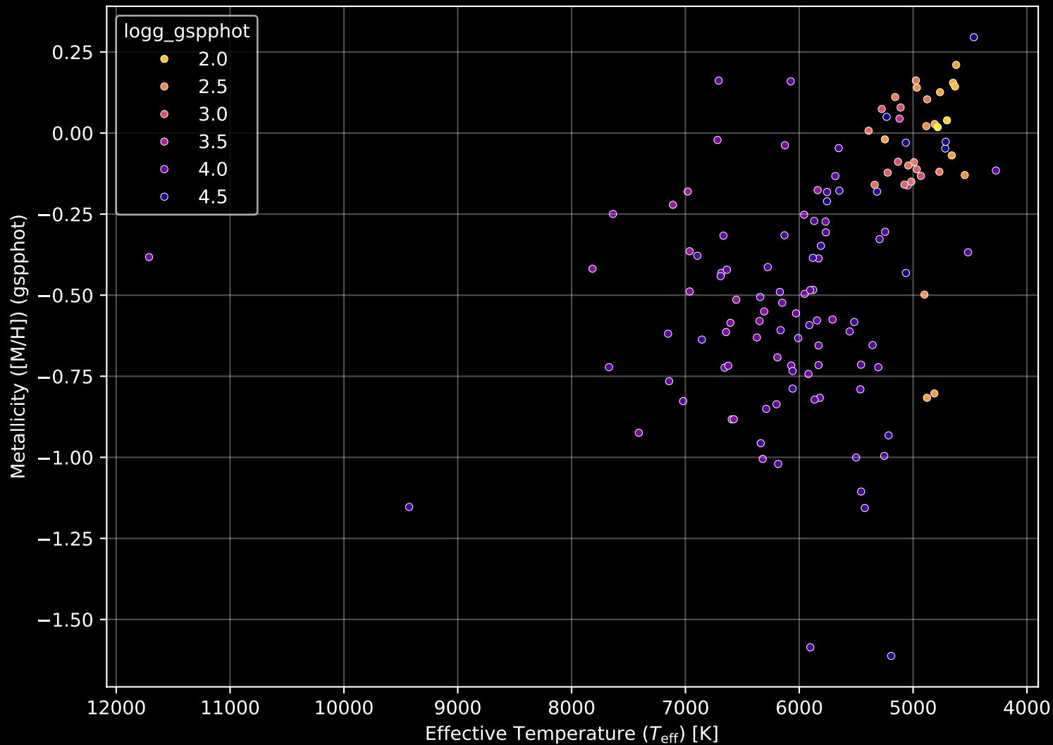
GALAH DR4 Field: [6790] Stellar Population Parameters (n= 131)
