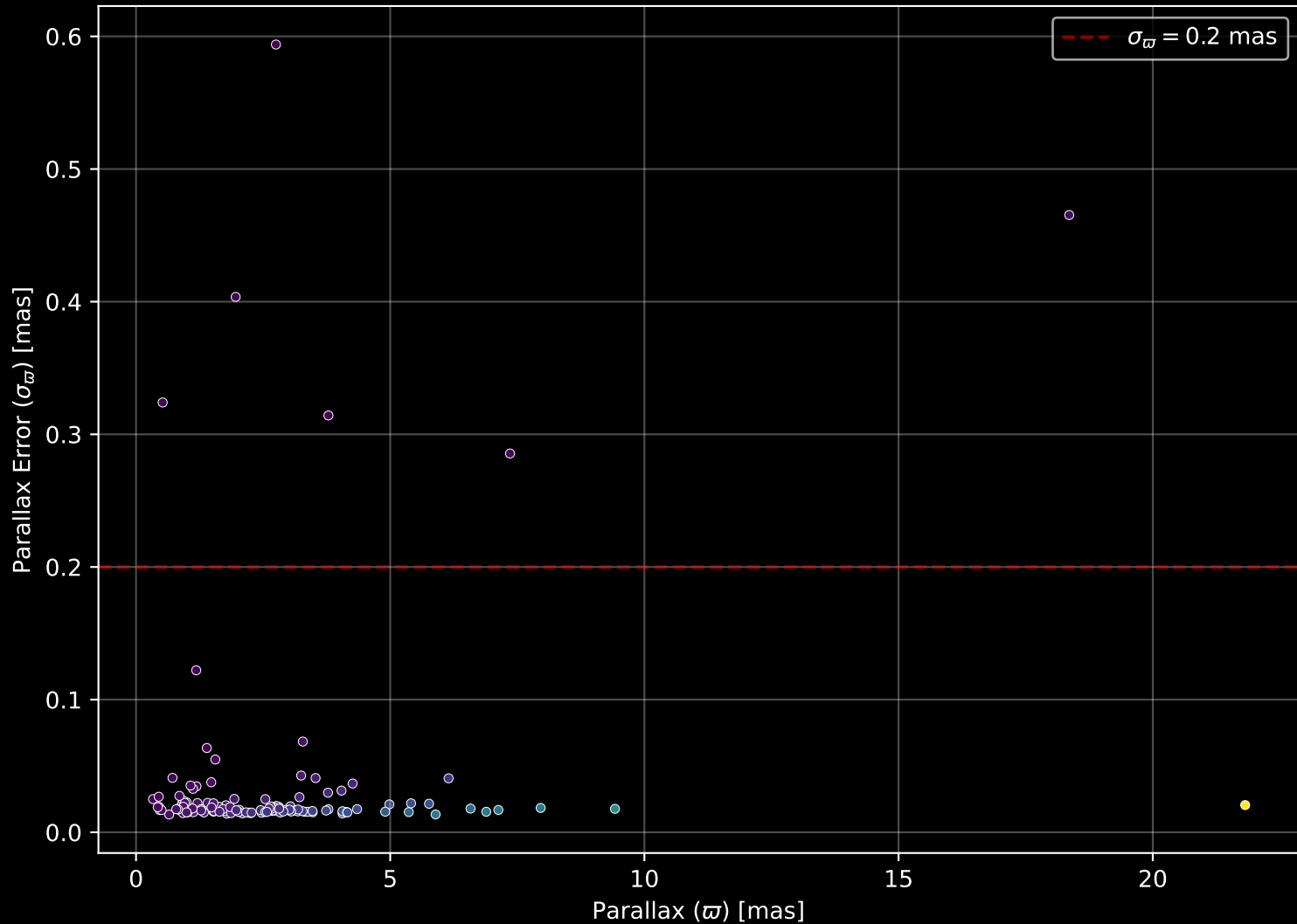
GALAH DR4 Field: [6790] Parallax Quality (n= 131)
