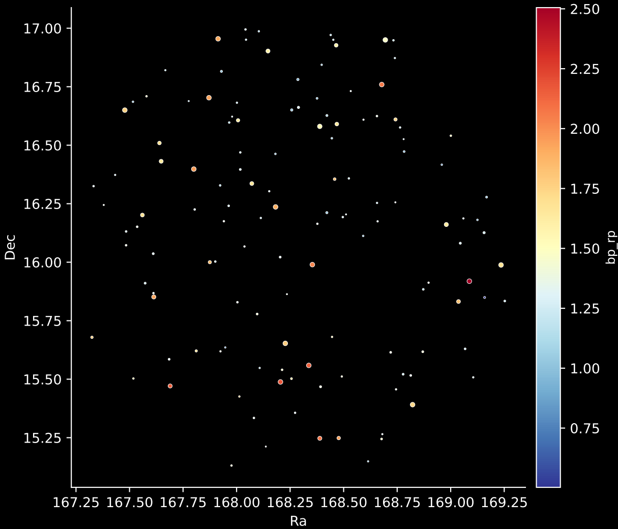
GALAH DR4 Field: [6790] Stars: 131
