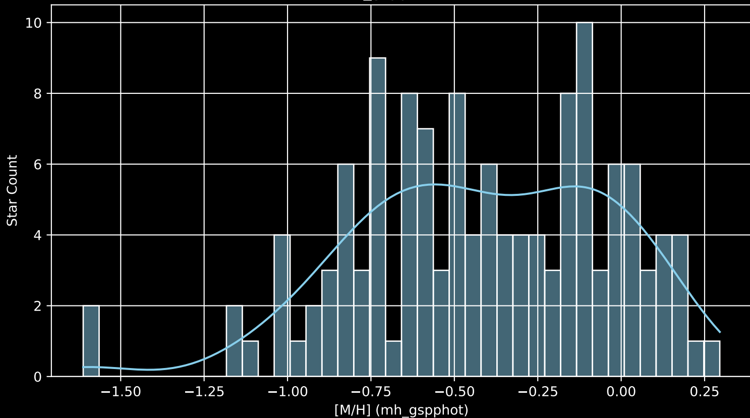
GALAH DR4 Field: [6790] [M/H] (mh_gspphot) (n= 131)
